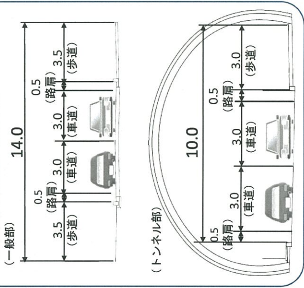
●標準的な断面図（単位：m）
